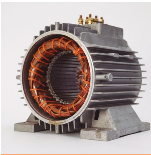
Bobinado de motores eléctricos
